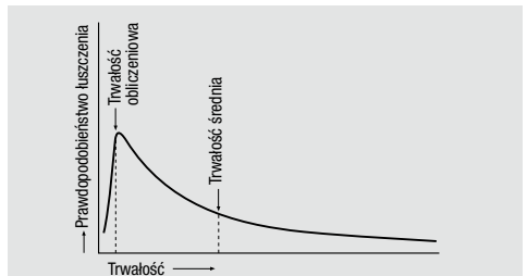
Rysunek 5.2 Prawdopodobieństwo zmęczenia a trwałość łożyska
