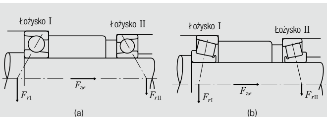
Rys. 5.12 Obciążenia w układzie przeciwnym podwójnym
