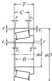
Rys. 7.2 Łożyska stożkowe
