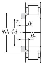
Piersienie kątowe typu L
