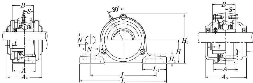
Typ z pokrywą przeciwpylową odlewaną przelotowa C-UCP...D1 nieprzelotowa CM-UCP...D1
