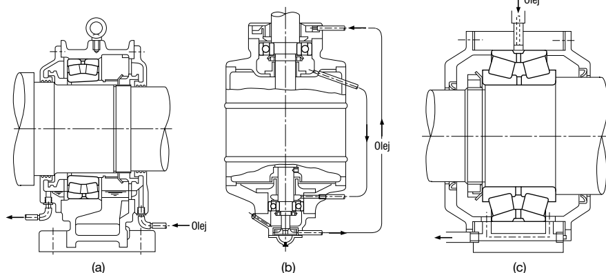
Rys.12.7 Smarowanie obiegowe
