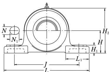
Typ z pokrywą przeciwpływową stalową tłoczoną przelotowa Z-UCP...D1 nieprzelotowa ZM-UCP...D1
