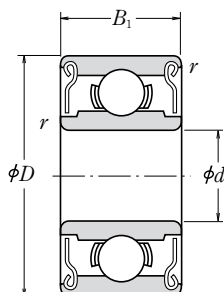
Typ z blaszką ZZ · ZJS
