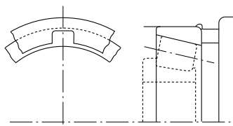
Rys. 14.11 Kanałki w oprawie łożyska stożkowego do założenia ściągnacza
