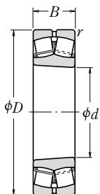
Otwór stożkowy
