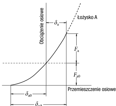
Rys. 10.5 Przemieszczenie osiowe przy napięciu wstępnym o stałej wartości
