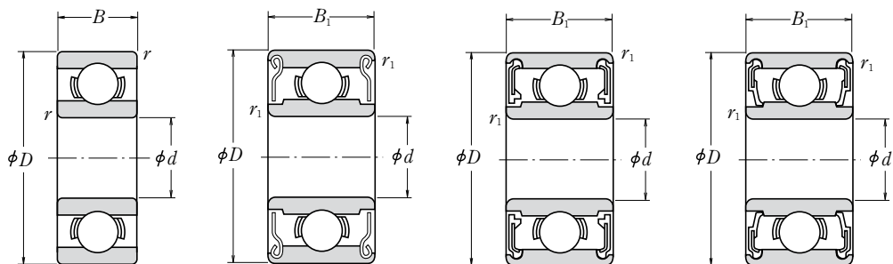
Typ z blaszką ZZ · ZZ1
