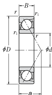
Pojedyncze
