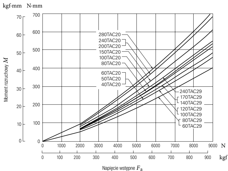
Rys.15.12 Napięcie wstępne oraz moment rozruchowy dla łożysk kulkowych skośnych wzdłużnych dwukierunkowych
