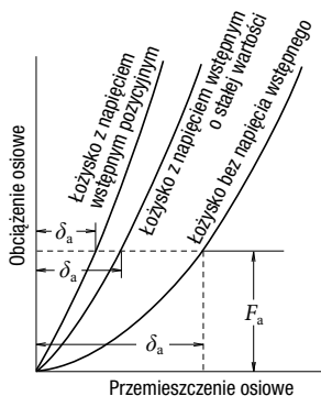
Rys. 10.6 Porównanie sztywności oraz metod napięcia wstępnego
