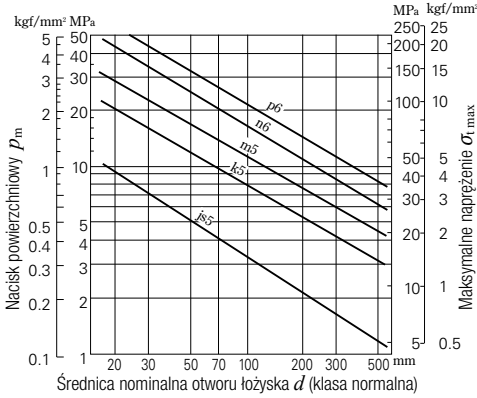
Rys. 15.5 Nacisk powierzchniowy p_m oraz maksymalne naprężenie \sigma_{t \max} dla wciśku średniego
