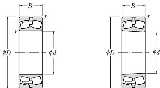
Otwór walcowy
