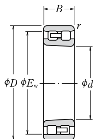
NN Otwór stożkowy
