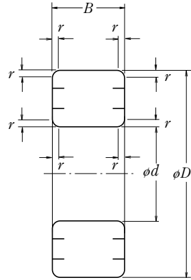
Rys. 7.1 Wymiary główne łożysk poprzecznych, kulkowych i wałeczkowych
