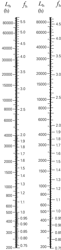
łożyska kulkowe
