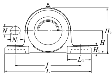
Typ z pokrywą przeciwpływową stalową tłoczoną przelotowa Z-UCP...D1 nieprzelotowa ZM-UCP...D1
