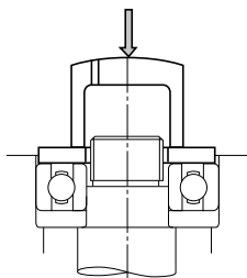
Rys. 14.2 Równoczesne wciskanie przy pomocy prasy pierścienia wewnętrznego i zewnętrznego
