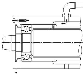
Rys. 12.9 Smarowanie mgłą olejową
