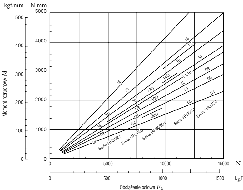
Rys. 15.10 Relacja pomiędzy obciążeniem osiowym a momentem rozruchowym łożysk stożkowych
