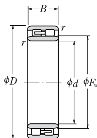
NNU Otwór walcowy
