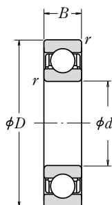
Typ otwarty
