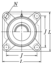
Typ z pokrywą przeciwpływową stalową tłoczoną przelotowa Z-UCF...D1 nieprzelotowa ZM-UCF...D1
