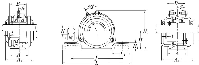
Typ z pokrywą przeciwpływową odlewaną przelotowa C-UCP...D1 nieprzelotowa CM-UCP...D1
