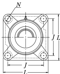
Typ z pokrywą przeciwpylową stalową tłoczoną przelotowa Z-UCF...D1 nieprzelotowa ZM-UCF...D1
