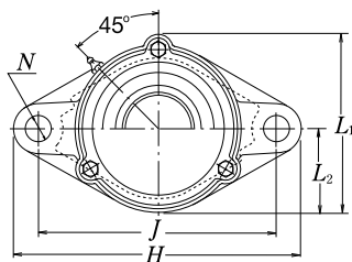
Typ z pokrywą przeciwpylową odlewaną przelotowa C-UCFL...D1 nieprzelotowa CM-UCFL...D1
