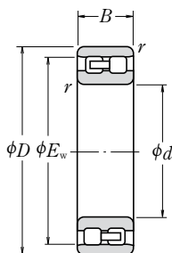
NN Otwór walcowy
