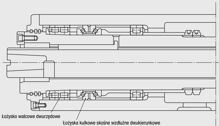
Przykład zastosowania łożyska kulkowego skośnego wzdluznego dwukierunkowego (wrzeczono glowne obrabiarki narzeczdziowej)
