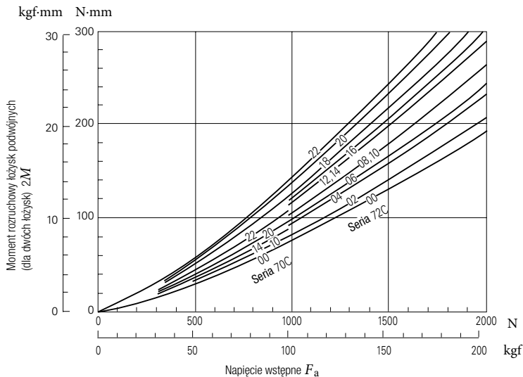
Rys. 15.11 Napięcie wstępne oraz moment rozruchowy dla łożysk kulkowych skośnych w układach „X” oraz „O” ( \alpha = 15^\circ )
