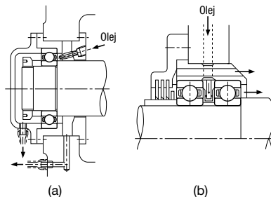
Rys. 12.8 Smarowanie strumieniowe
