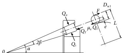
Rys. 15.9 Relacja pomiędzy e oraz \beta
