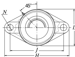
Typ z pokrywą przeciwpylową stalową tłoczoną przelotowa Z-UCFL...D1 nieprzelotowa ZM-UCFL...D1
