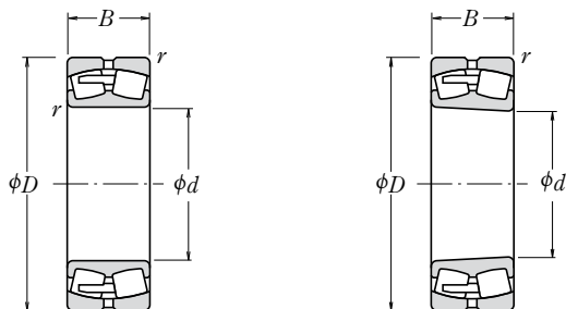
Otwór walcowy
