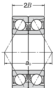
W układzie 0 DB
