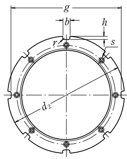
Nakrętka z podkładką kształtowaną
