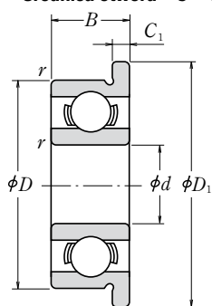
Typ otwarty
