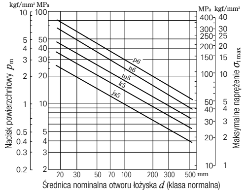
Rys. 15.6 Nacisk powierzchniowy p_m oraz maksymalne naprężenie \sigma_{t \max} dla wciśku maksymalnego
