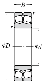
Otwór walcowy
