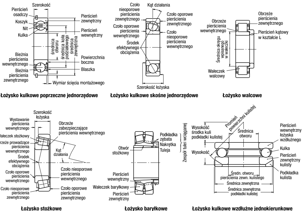
Rysunek 1.1 Terminologia dla części łożyskowych
