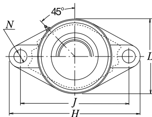
Typ z pokrywą przeciwpływową stalową tłoczoną przelotowa Z-UCFL...D1 nieprzelotowa ZM-UCFL...D1
