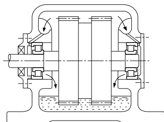
Rys. 12.6 Smarowanie rozbryzgowie
